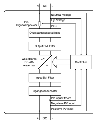
Enphase IQ8X Microinverter
