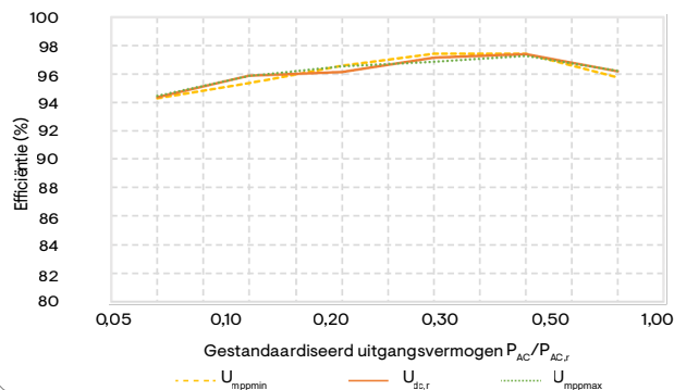
IQ8X Microinverter efficiëntiecurve
