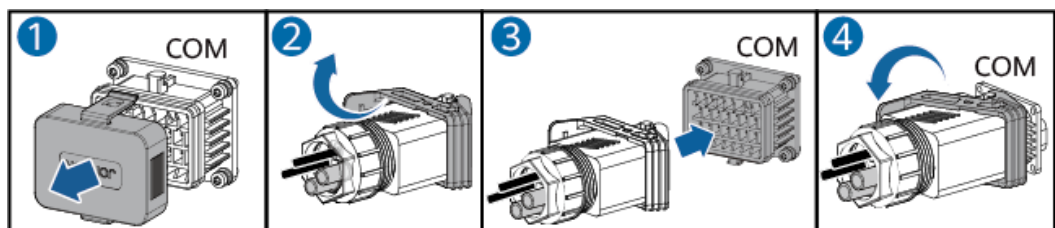
Abbildung 5-47 Sichern des Signalkabelsteckverbinders
