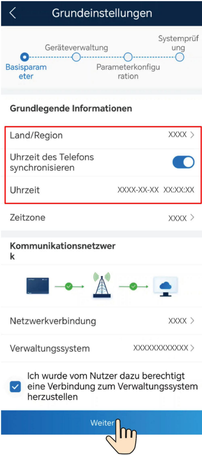
Abbildung 7-6 Basisparameter (am Beispiel der Vernetzung mit SmartLogger5000B)
