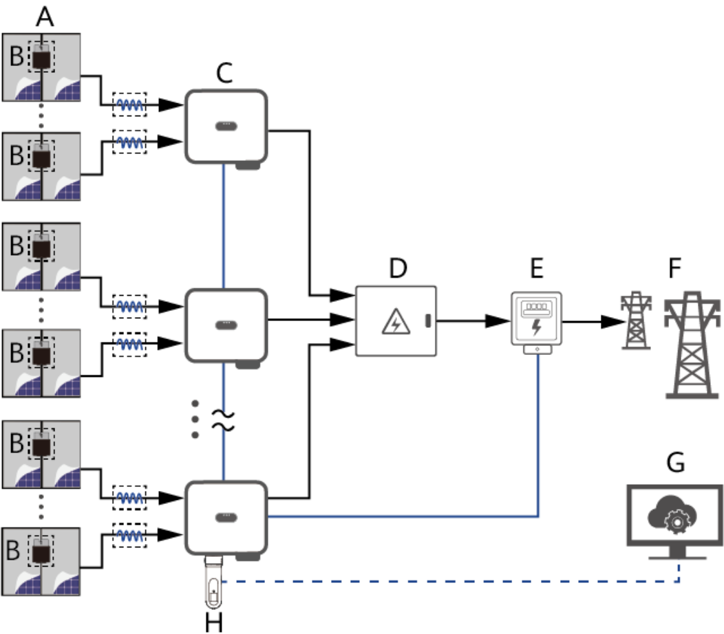
Abbildung 2-3 RS485-Vernetzung (Dongle)
