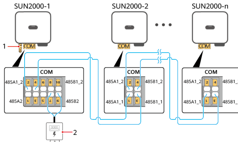
Abbildung 5-29 Smart Dongle-Vernetzung
