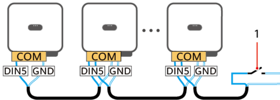
Abbildung 5-45 Anschließen von kaskadierten Wechselrichtern an den NS-Schutzschalter
