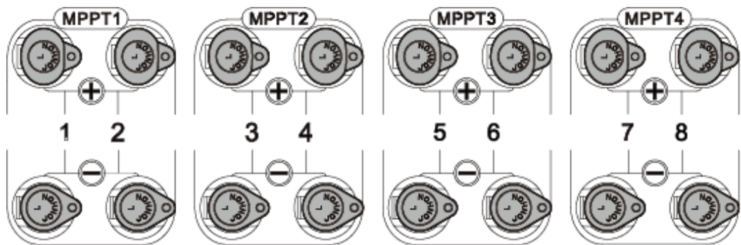
Abbildung 5-12 DC-Eingangsklemmen
