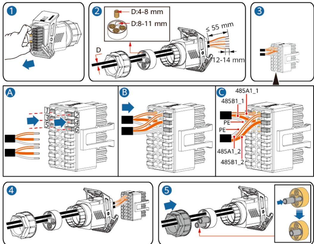
Abbildung 5-31 Kabelmontage
