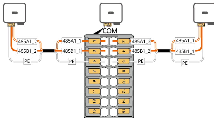
Abbildung 5-30 Kabelverbindung
