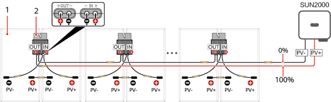
Abbildung 8-2 Definition des Prozentsatzes der Kurzschlussposition (Optimierer konfiguriert)
