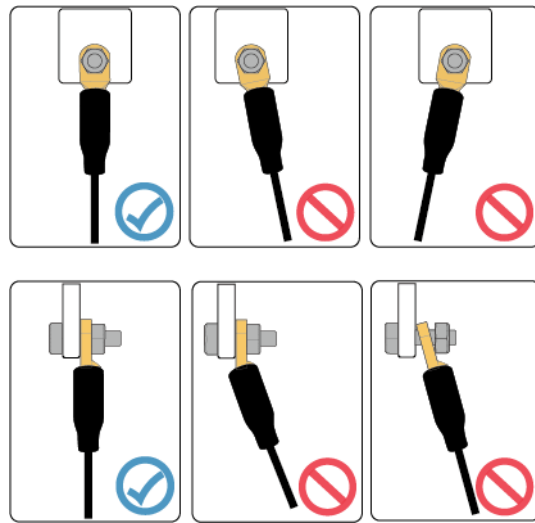
Abbildung 5-11 Verdrahtungsanforderungen
