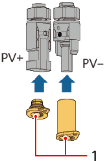
Abbildung 5-22 Verschlussstopfen
