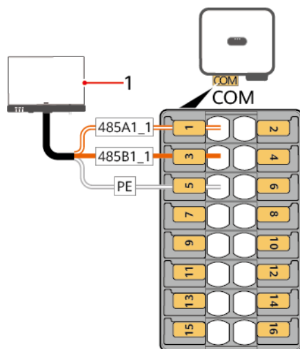
Abbildung 5-33 Kabelverbindung
