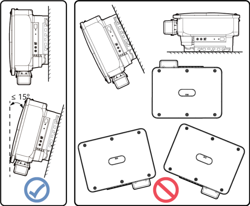
Abbildung 4-9 Installationswinkel
