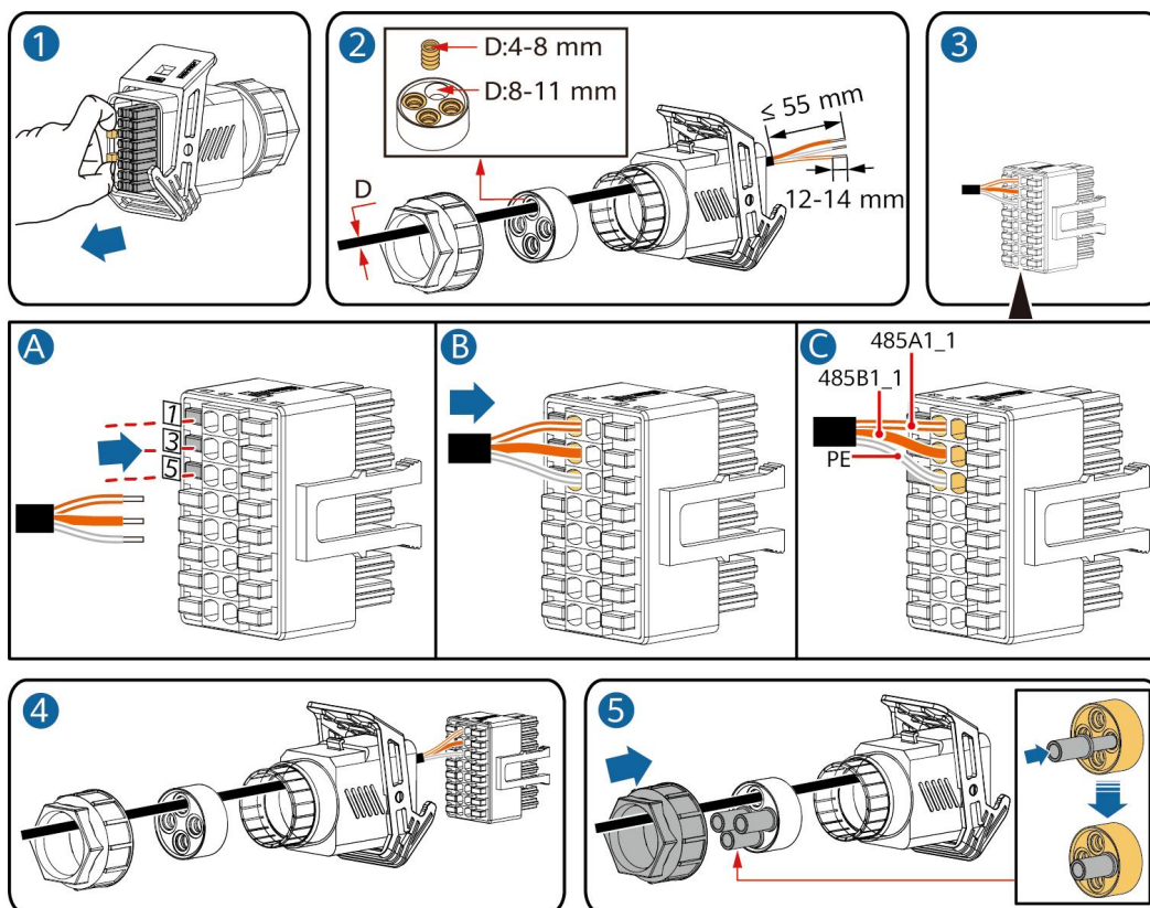
Abbildung 5-34 Kabelmontage
