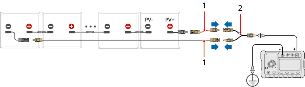
Abbildung 5-19 Messung des Isolationswiderstands des Verlängerungskabels
