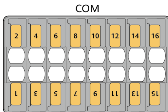
Abbildung 5-27 Pin-Belegung
