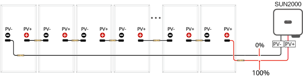
Abbildung 8-3 Definition des Prozentsatzes der Kurzschlussposition (Optimierer nicht konfiguriert)
