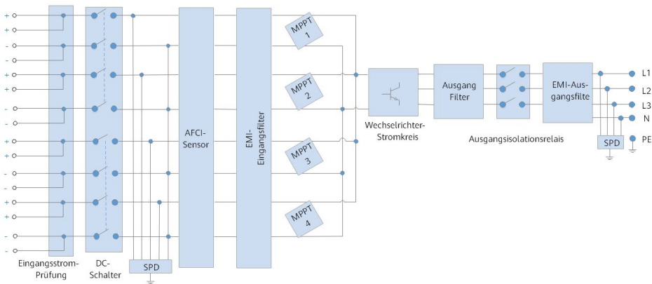
Abbildung 2-7 Schematisches Diagramm
