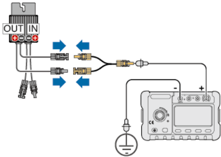
Abbildung 5-16 Messung des Isolationswiderstands eines Optimierers
