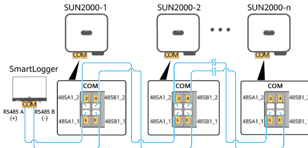
Abbildung 5-28 SmartLogger-Vernetzung
