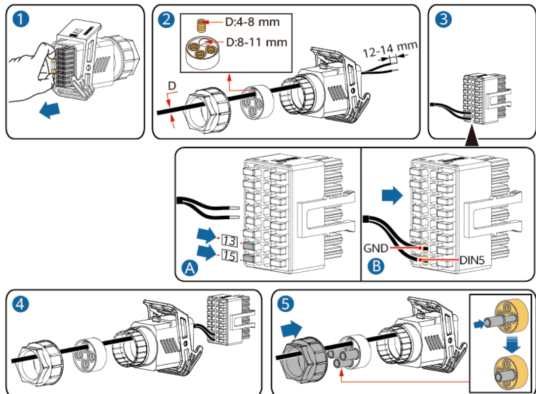
Abbildung 5-43 Kabelmontage
