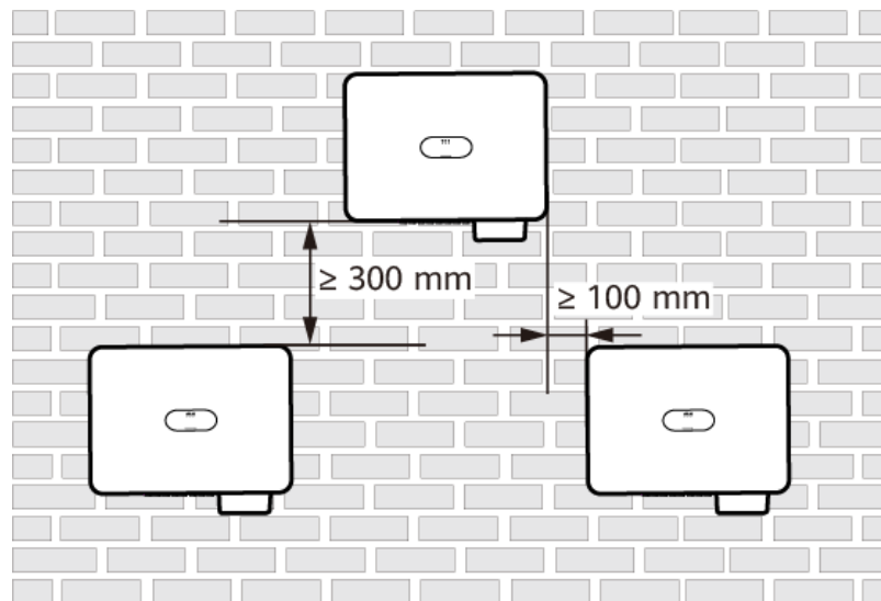
Abbildung 4-5 Zweistufige Dreiecksmontage (empfohlen)
