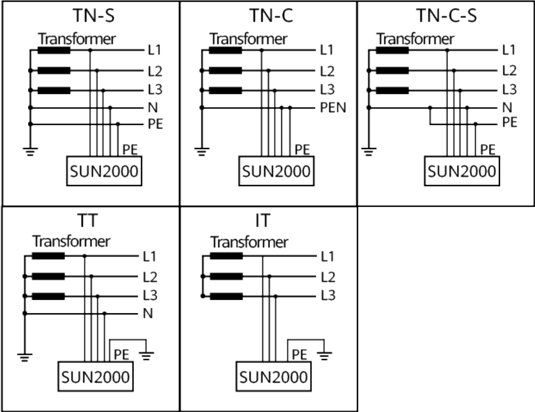
Afbeelding2-3 Aardingssystemen
