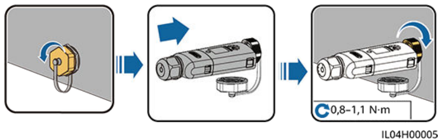
Afbeelding5-16 De WLAN-FE Smart Dongle installeren (WLAN-communicatie)
