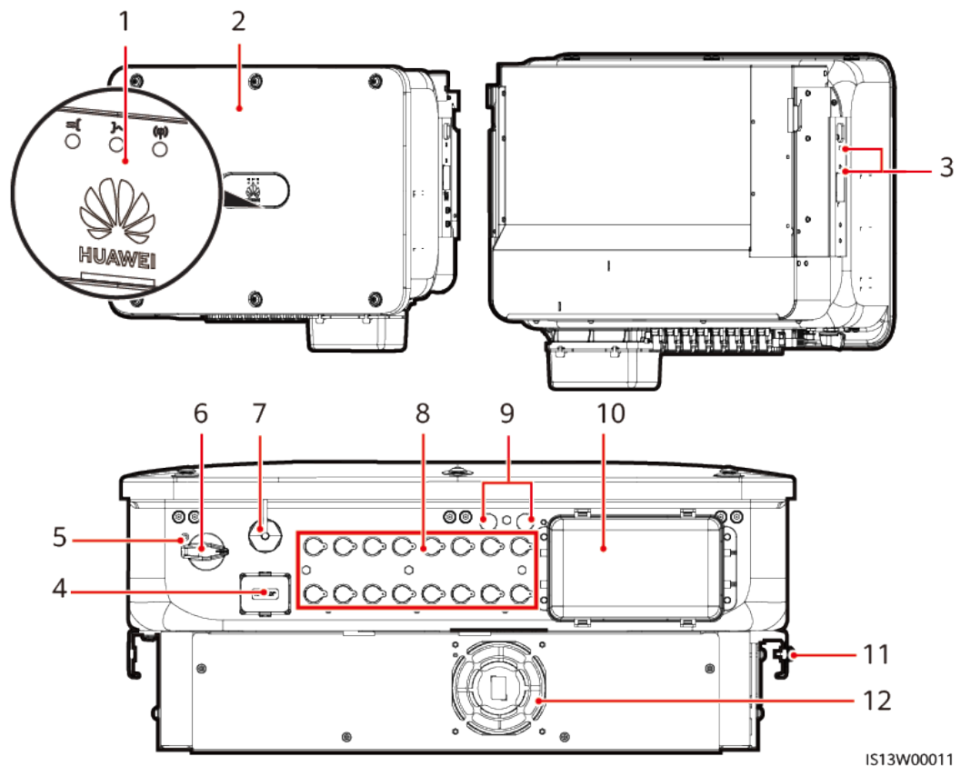
Afbeelding 2-4 Uiterlijke kenmerken
