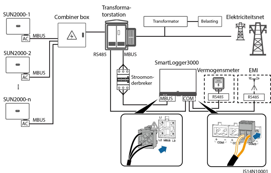
Afbeelding5-22 MBUS-communicatie (scenario voor nutsbedrijven)
