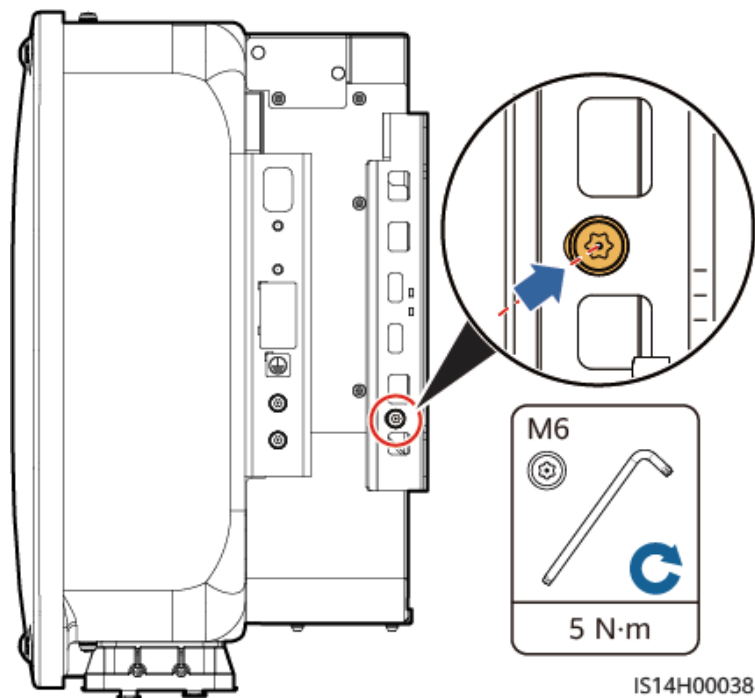
Afbeelding4-18 Moeren vastdraaien
