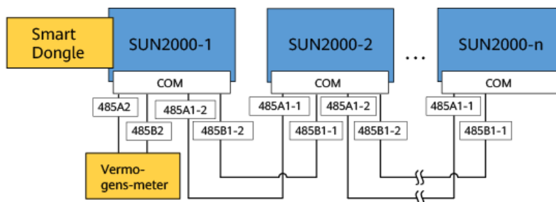
Afbeelding5-20 Smart Dongle-netwerk
