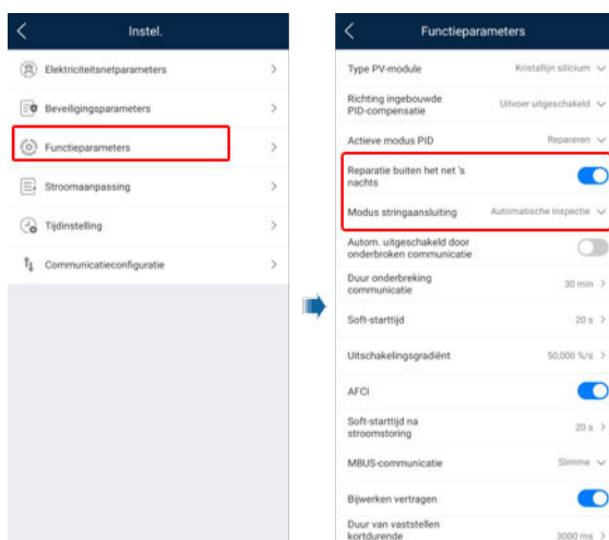
AfbeeldingC-1 PID-onderdrukkingsparameters instellen
