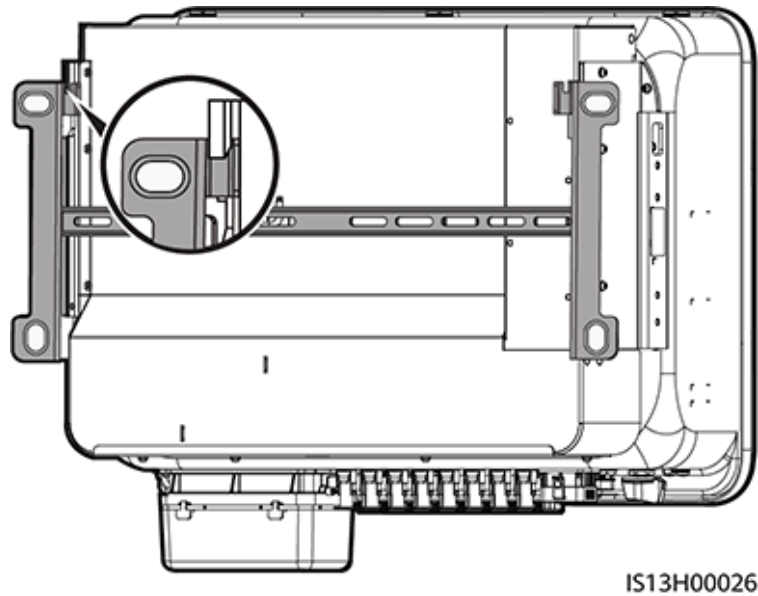
Afbeelding4-17 De omvormer installeren
