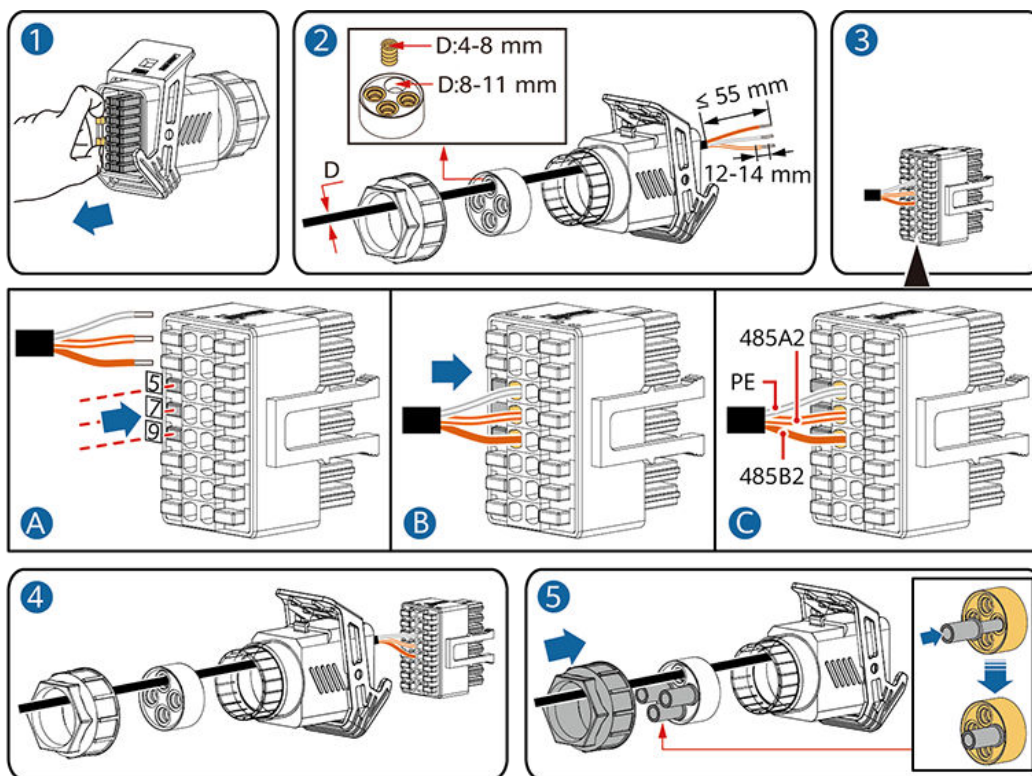
Afbeelding5-26 De kabel installeren
