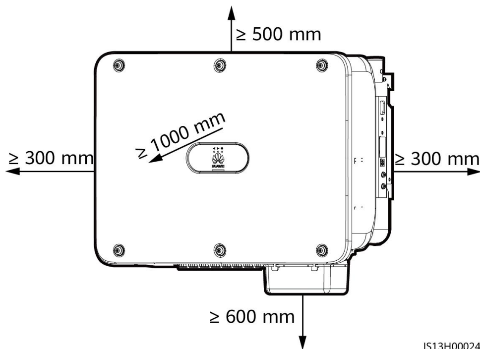
Afbeelding4-2 Vrije ruimte
