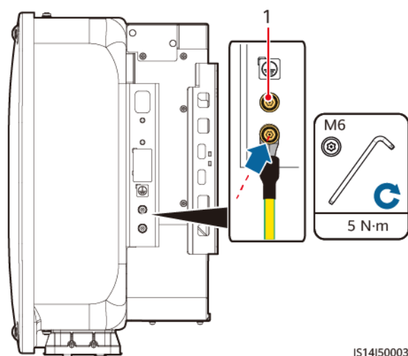
Afbeelding5-3 Een PE-kabel aansluiten
