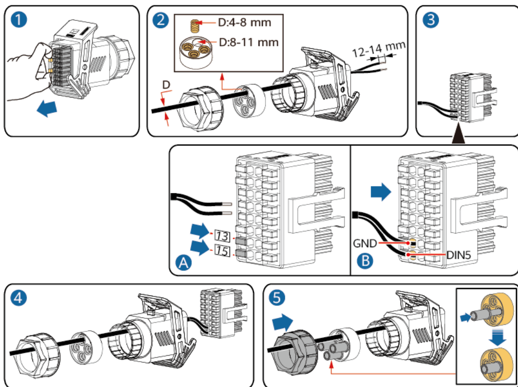
Afbeelding5-30 De kabel installeren
