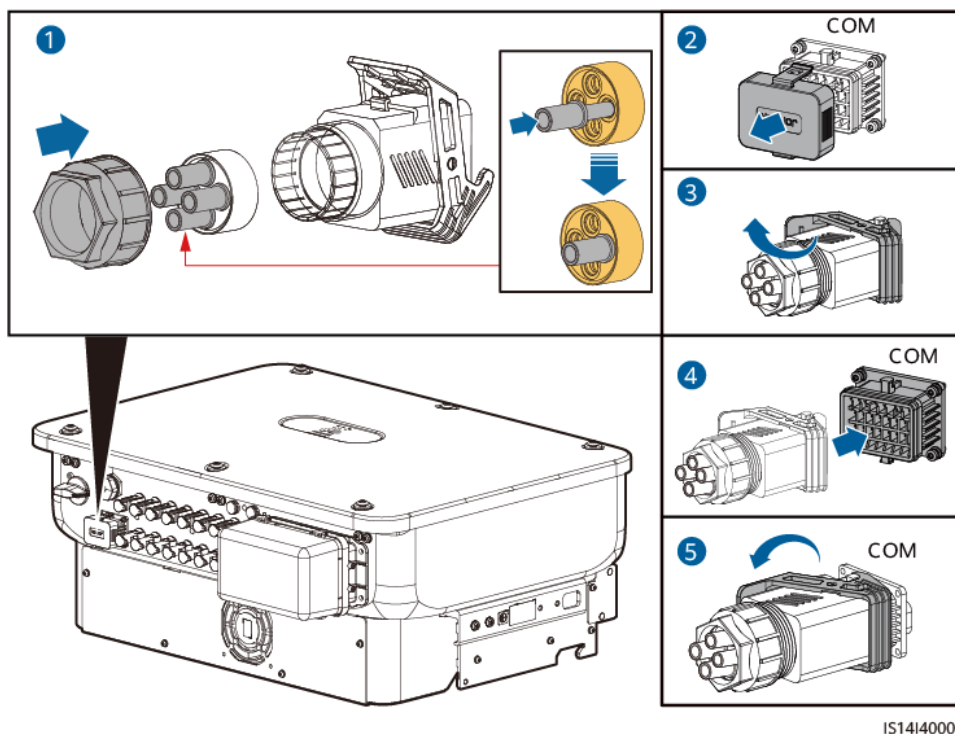
Afbeelding5-19 De aansluiting van de signaalkabel aansluiten
