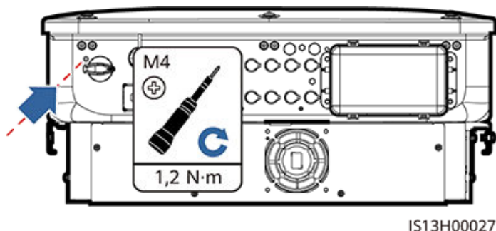
Afbeelding8-1 De borgschroef van de DC-schakelaar installeren
