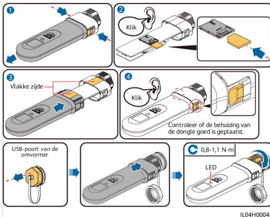
Afbeelding5-15 De 4G Smart Dongle (SDongleB-06) installeren
