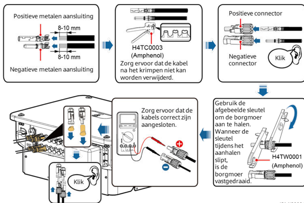
Afbeelding5-13 DC-voedingskabels aansluiten
