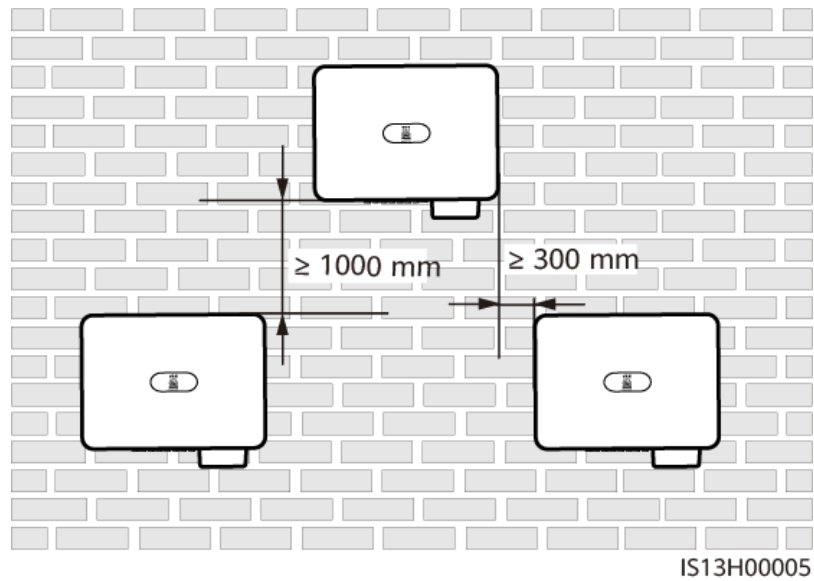
Afbeelding4-4 Installatie in driehoek met twee lagen (niet aanbevolen)
