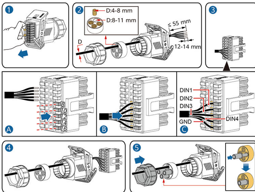
Afbeelding5-28 De kabel aansluiten
