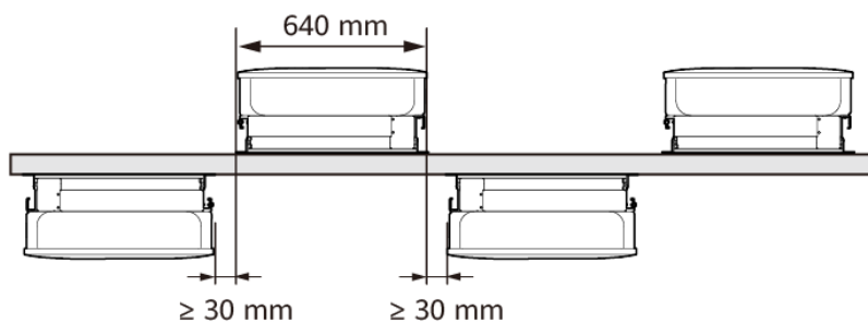
Afbeelding4-8 Rug-aan-rug verspringende installatie op een steun (aanbevolen)
