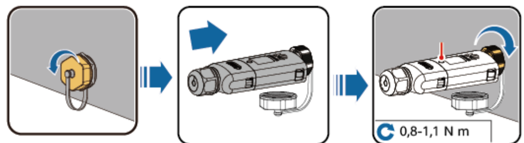
Abbildung 5-20 Installieren des WLAN-FE Smart Dongle (SDongleA-05 für das WLAN-Kommunikationsszenario)
