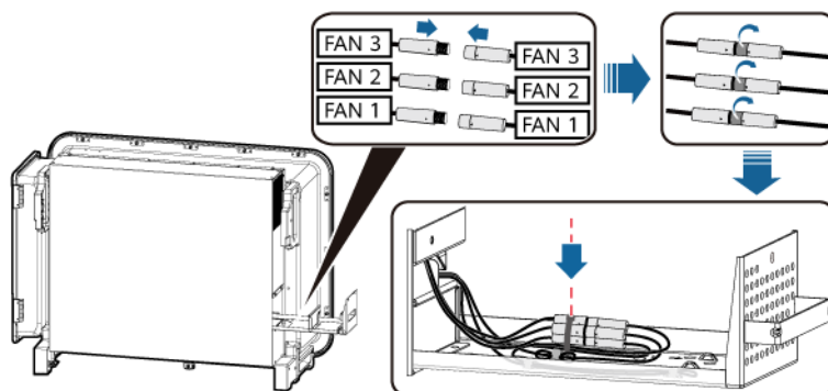
Abbildung 8-14 Binden der Kabel
