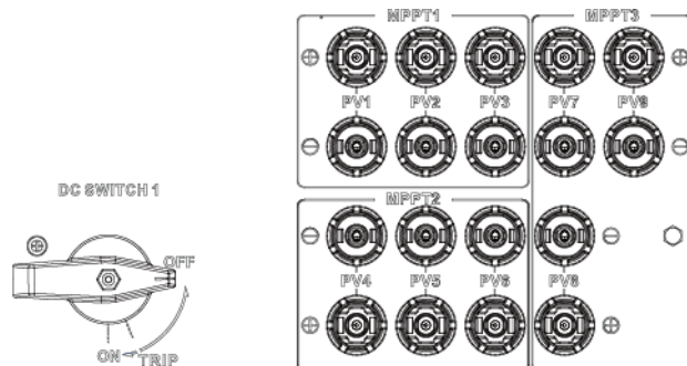
Abbildung 5-10 Von DC SWITCH 1 gesteuerte DC-Klemmen
