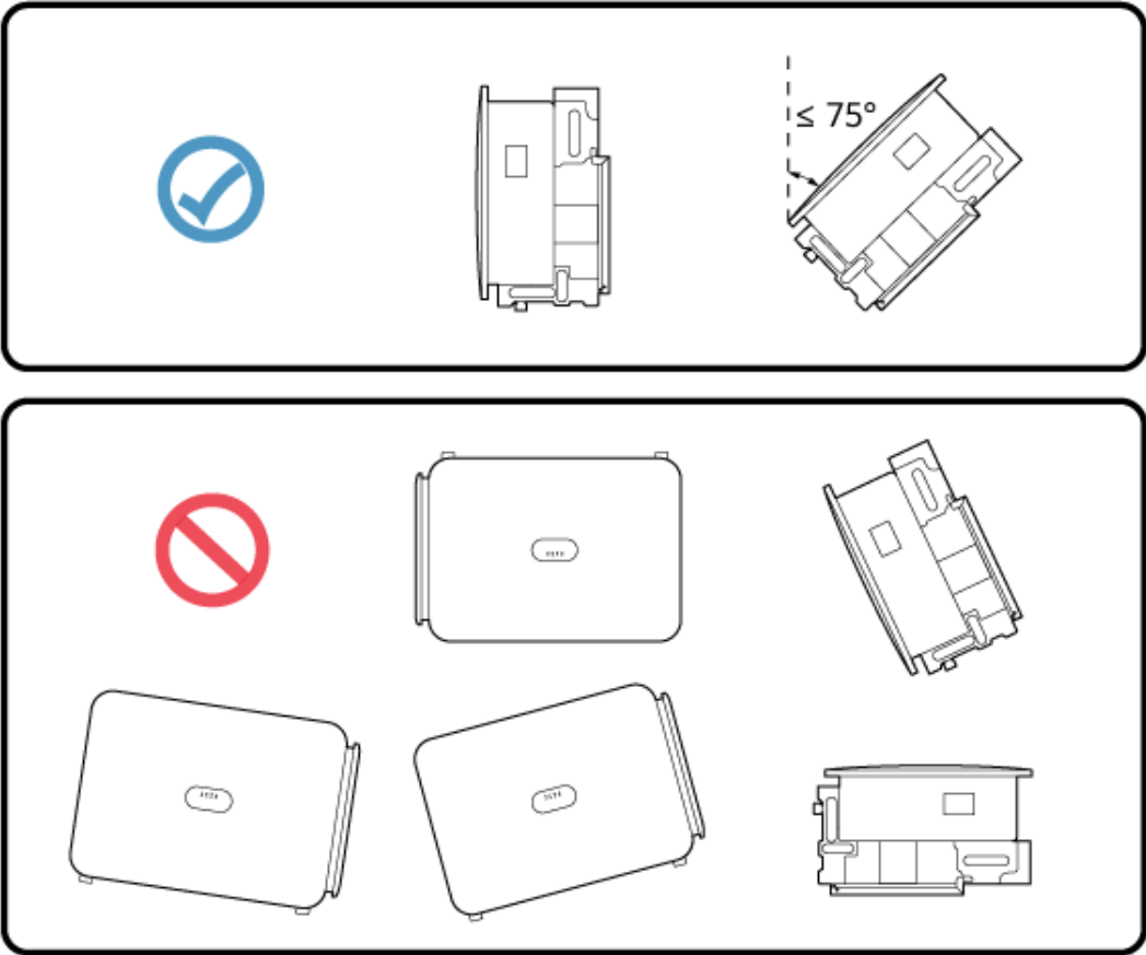
Abbildung 4-8 Installationswinkel
