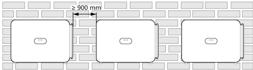
Abbildung 4-4 Horizontaler Installationsmodus (empfohlen)
