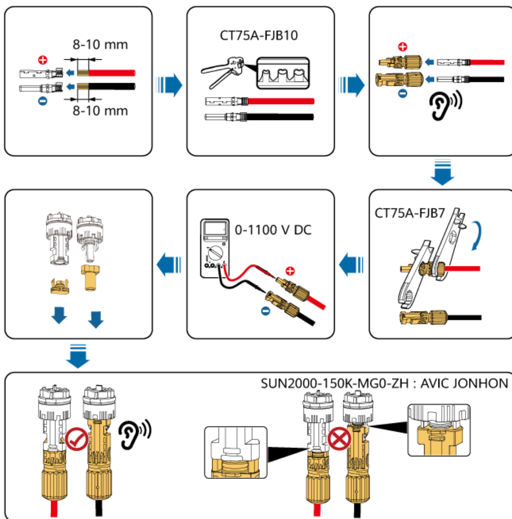
Abbildung 5-14 Anschließen der DC-Eingangsstromkabel (AVIC JONHON)
