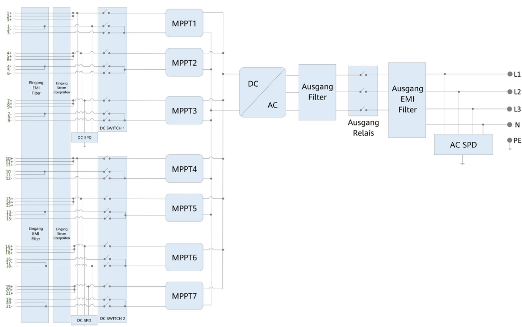
Abbildung 2-9 Stromlaufplan
