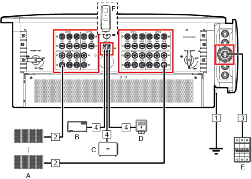
Abbildung 5-1 Kabelverbindungen (konfigurieren Sie die Komponenten im gestrichelten Kästchen nach Bedarf)
