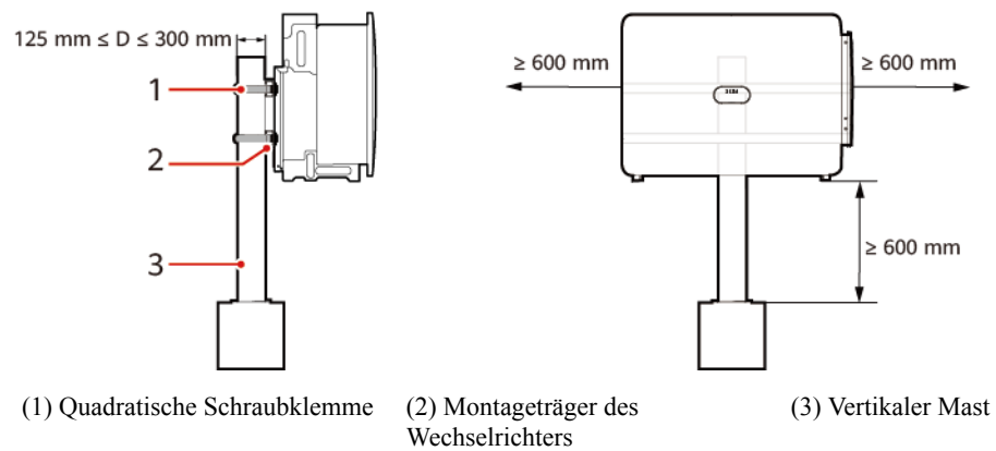
Abbildung 4-18 Installation mit Mastschelle
