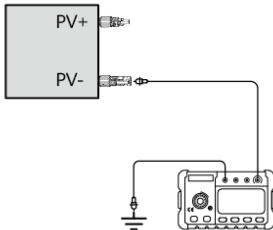
Abbildung 5-12 Prüfung des Isolationswiderstands
