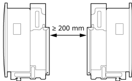
Abbildung 4-6 Installation Rückseite-an-Rückseite (empfohlen)
