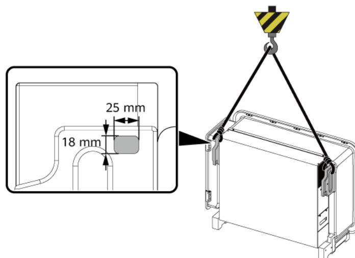
Abbildung 4-11 Heben
