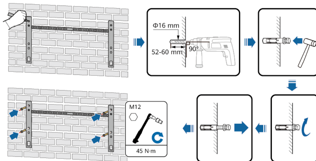
Abbildung 4-16 Einsetzen eines Spreizdübels
