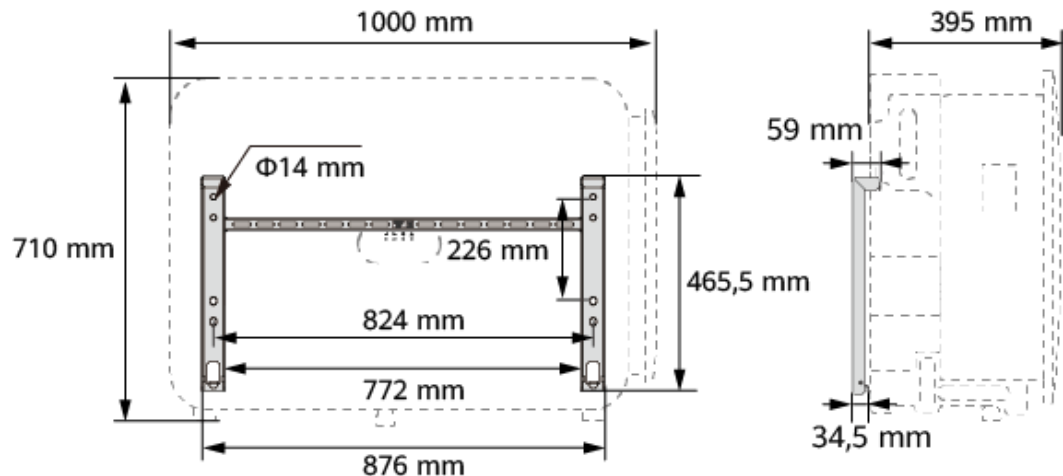
Abbildung 4-2 Abmessungen
