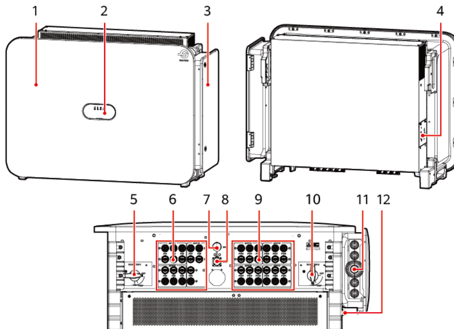
Abbildung 2-7 Erscheinungsbild
