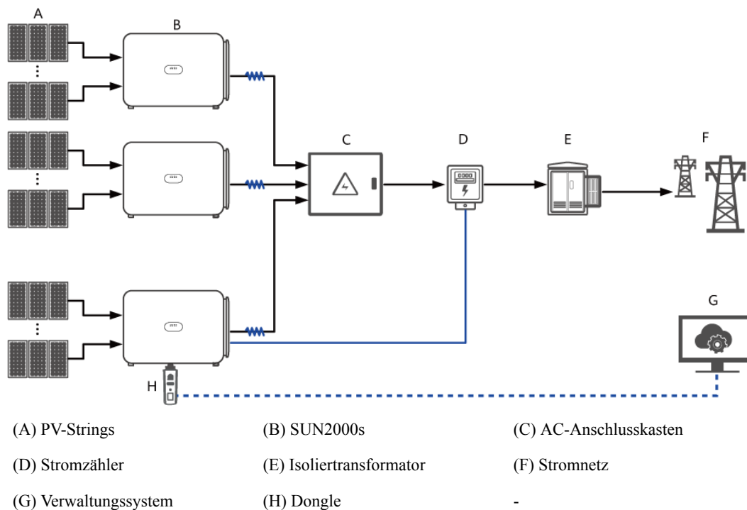
Abbildung 2-5 MBUS-Vernetzungsanwendung (Dongle)
