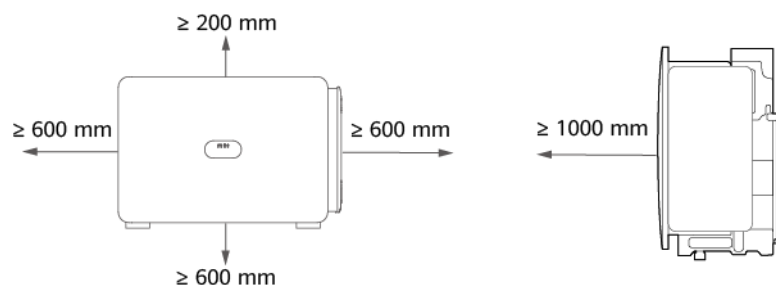
Abbildung 4-3 Abstände
