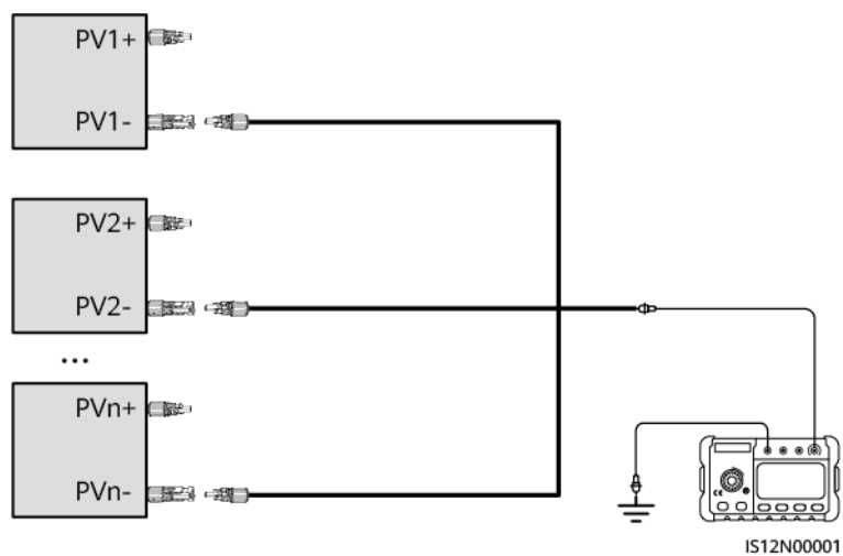
Abbildung 5-13 Messung des Isolationswiderstands aller PV-Kabel
