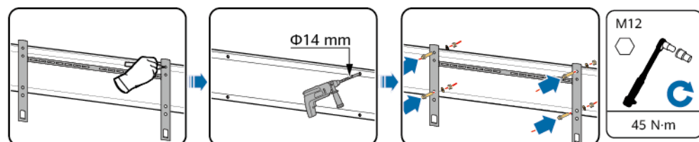
Abbildung 4-13 Anbringen der Montagehalterung
