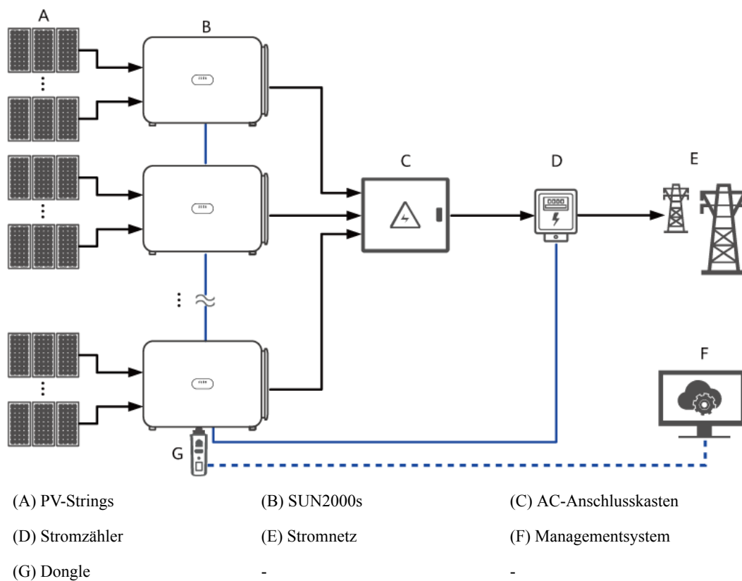
Abbildung 2-3 RS485-Vernetzungsanwendung (Dongle)
