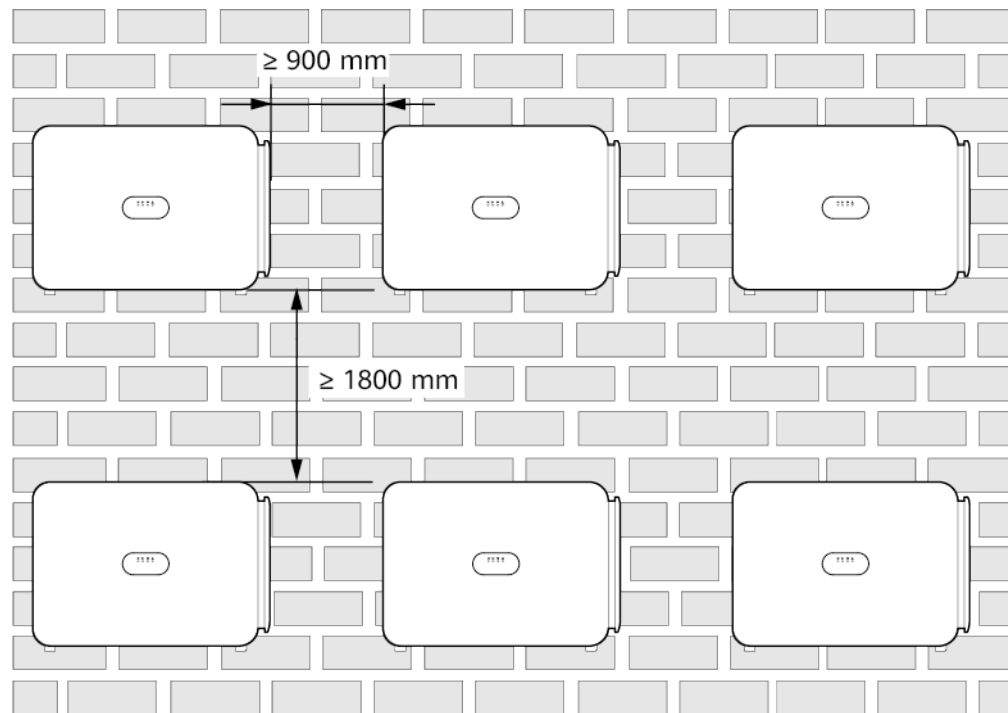
Abbildung 4-7 Gestapelte Montagemethode (nicht empfohlen)
