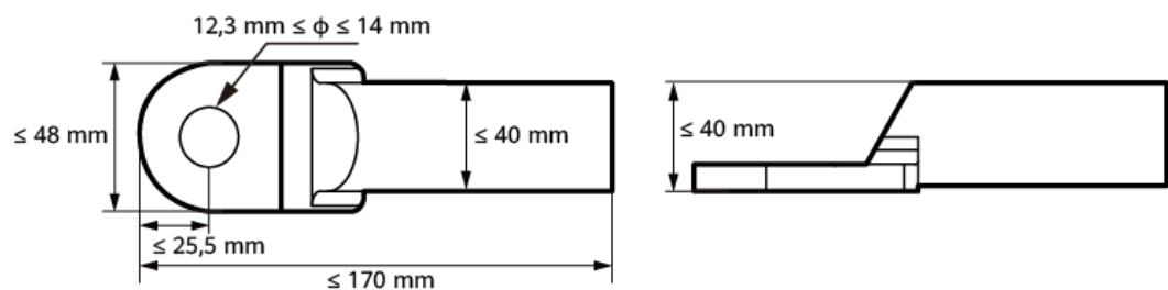
Abbildung 5-5 Spezifikationen der gekrimpten OT/DT-Klemme
