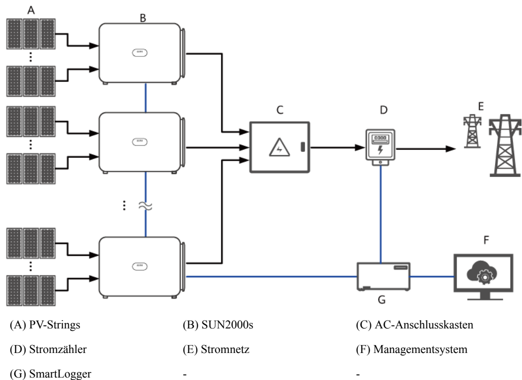
Abbildung 2-2 RS485-Vernetzungsanwendung (SmartLogger)
