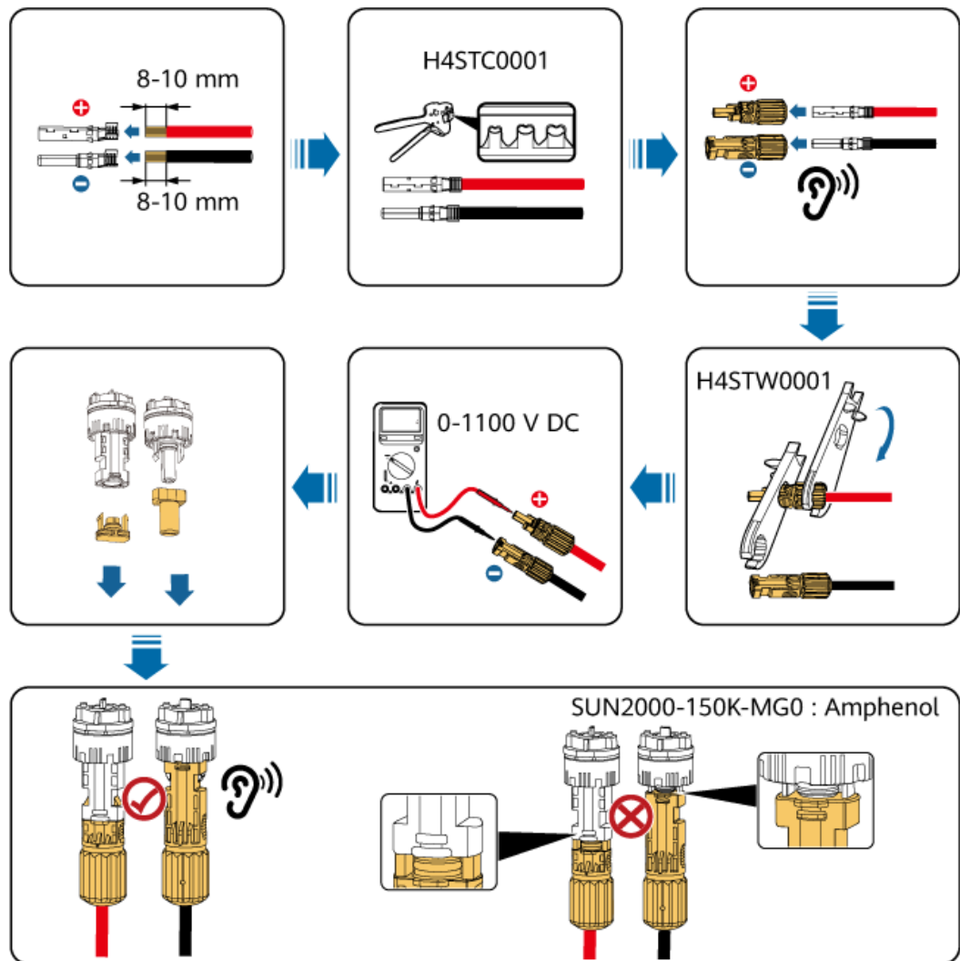
Abbildung 5-15 Anschließen der DC-Eingangsstromkabel (Amphenol)
