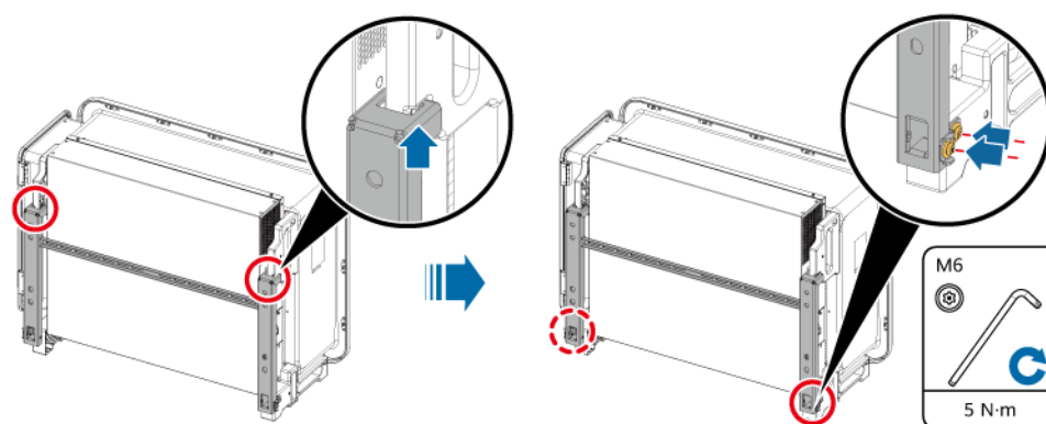
Abbildung 4-17 Sicherung des Wechselrichters
