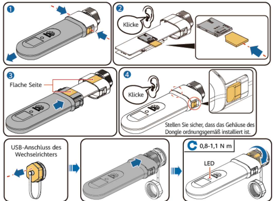
Abbildung 5-19 Installation des 4G Smart Dongle (SDongleB-06)
