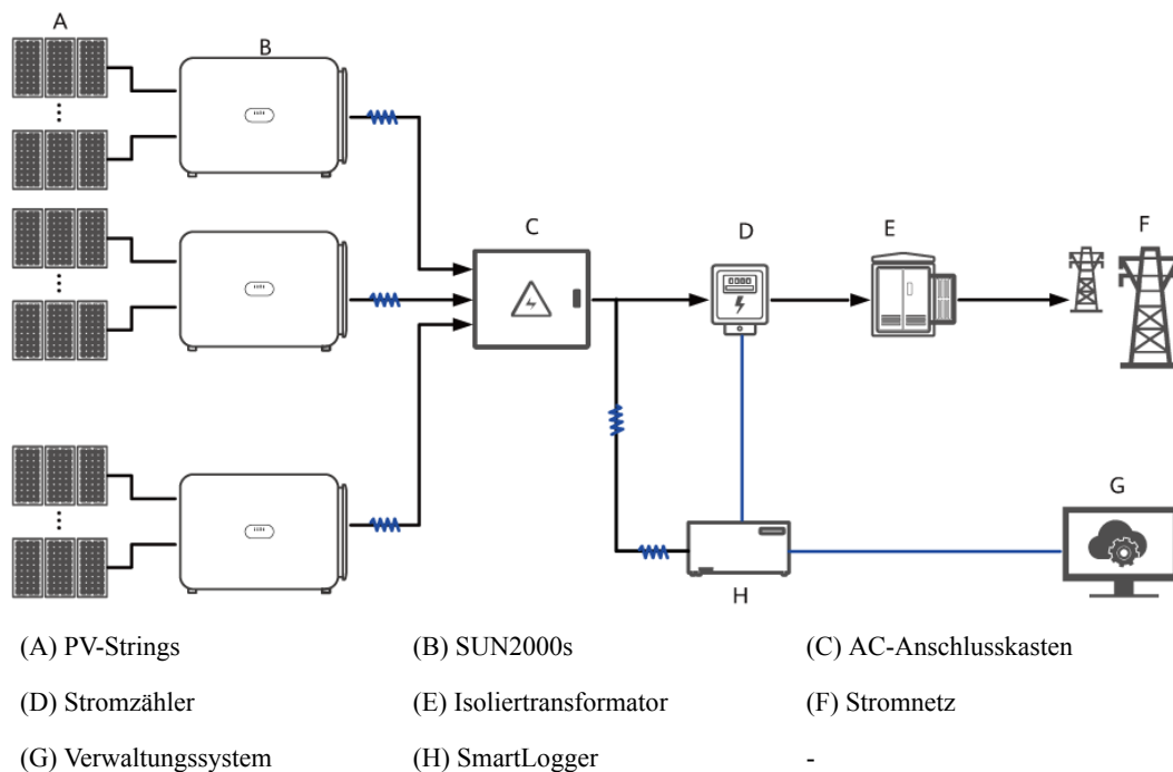
Abbildung 2-4 MBUS-Vernetzungsanwendung (SmartLogger)
