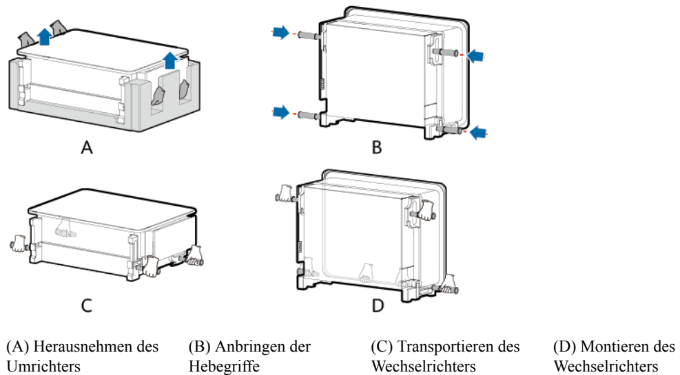
Abbildung 4-10 Hebepositionen
