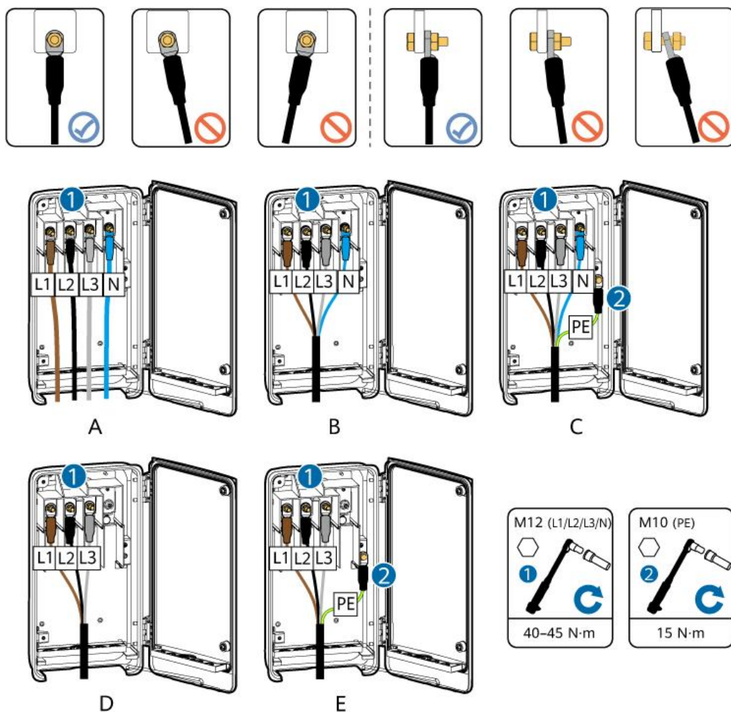
Abbildung 5-6 Kabelverbindung
