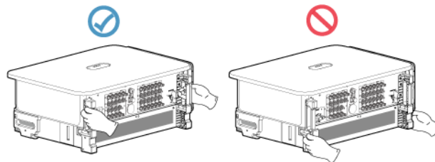
Abbildung 4-10 Hebepositionen
