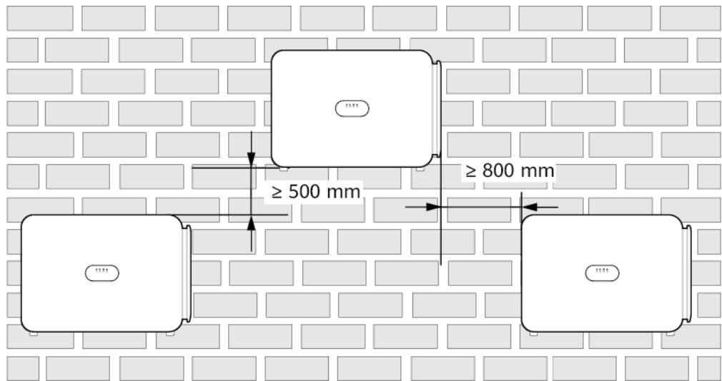
Abbildung 4-5 Dreiecks-Montagemethode (empfohlen)
