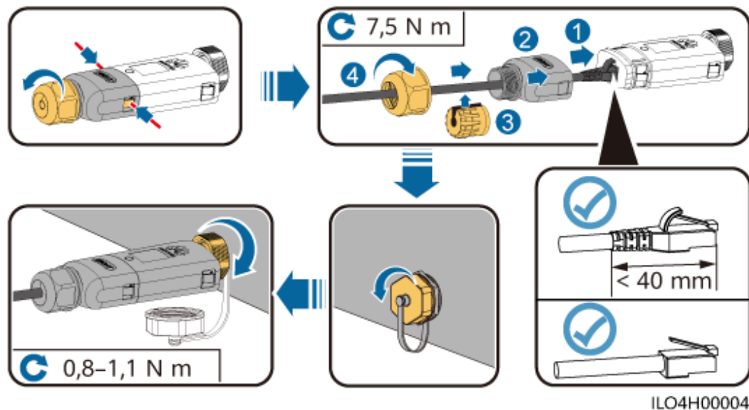
Abbildung 5-21 Installation des WLAN-FE Smart Dongle (SDongleA-05 für das FE-Kommunikationsszenario)
