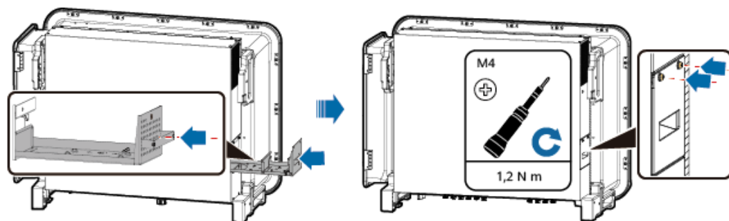
Abbildung 8-15 Wiedereinbau der Lüfterablage
