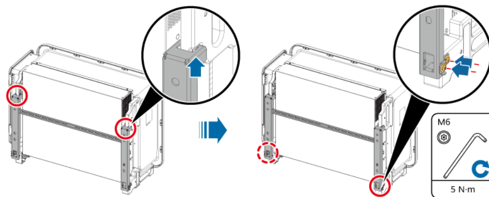
Abbildung 4-14 Sicherung des Wechselrichters
