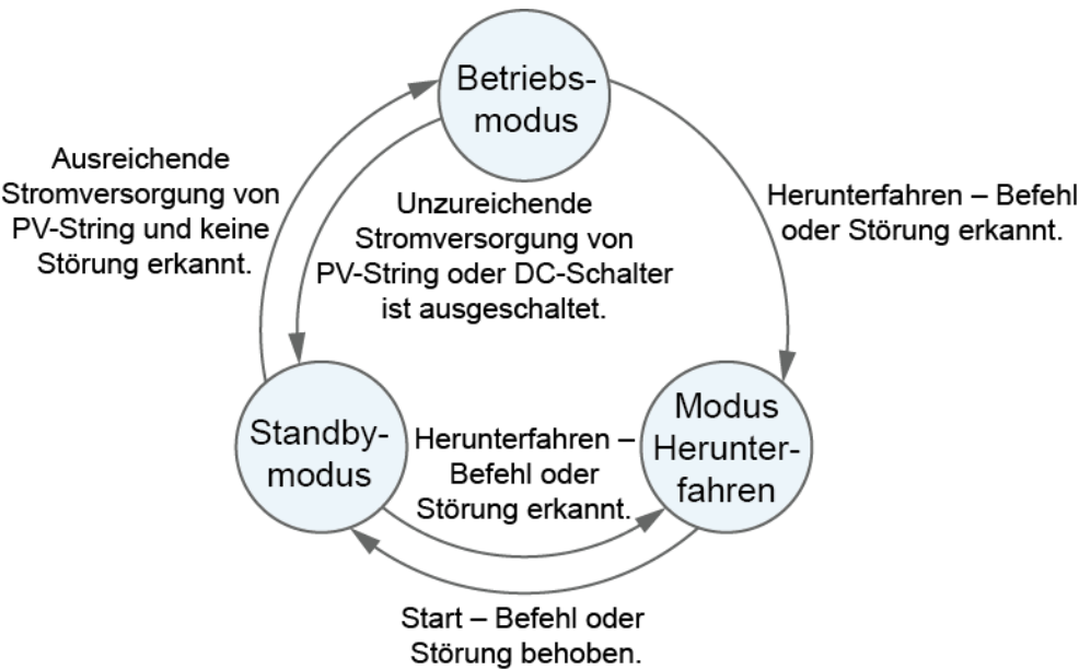
Abbildung 2-10 Arbeitsmodi
