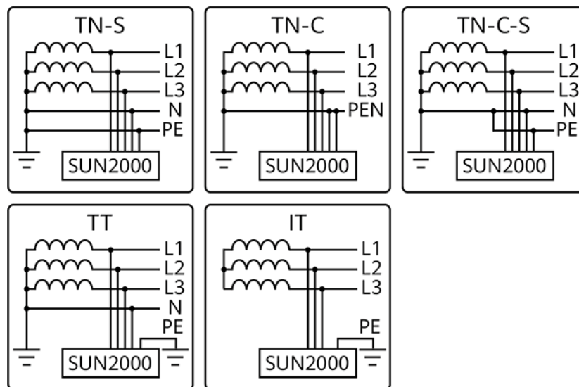
Abbildung 2-6 Erdungssysteme
