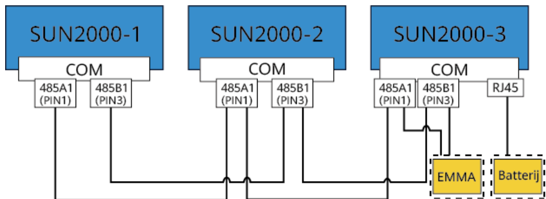
Afbeelding5-16 EMMA-netwerk (de onderdelen in kaders met een stippellijn zijn optioneel)
