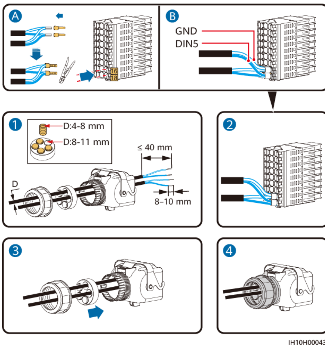
Afbeelding5-39 Kabels installeren
