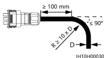
Afbeelding5-6 Bekabelingsvereisten
