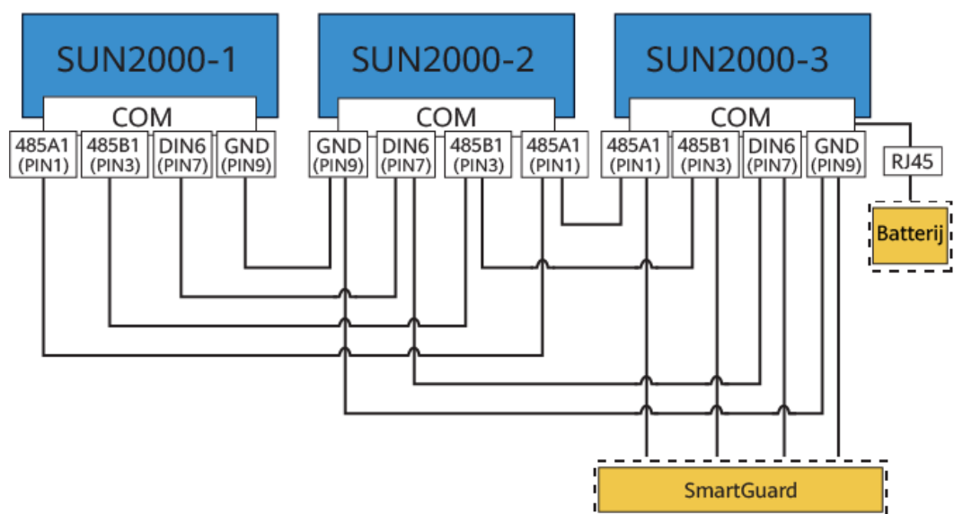
Afbeelding5-17 SmartGuard-netwerk (de onderdelen in kaders met een stippellijn rond zijn optioneel)
