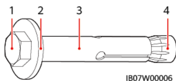
Afbeelding4-7 Structuurschema keilbouten
