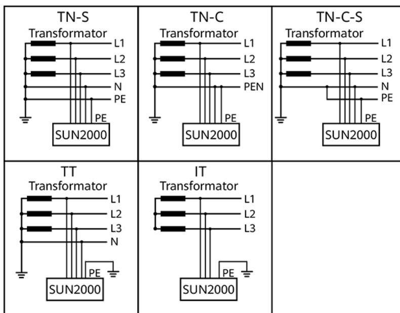
Abbildung 2-6 Unterstützte Stromnetze
