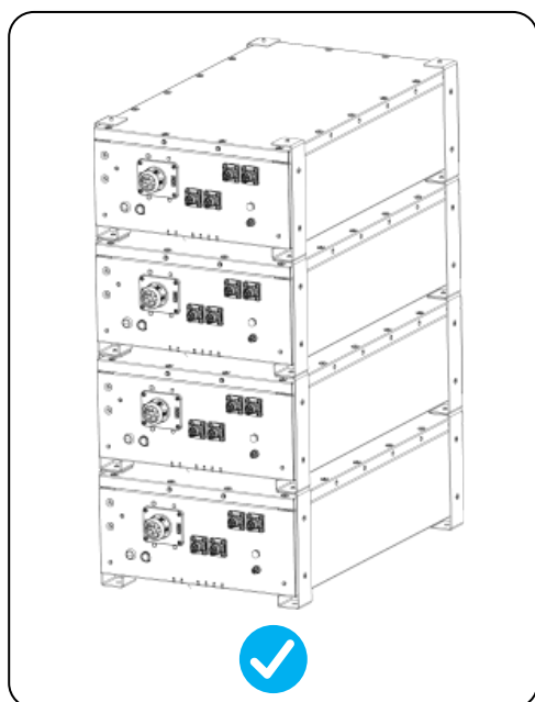
Stapeld door eenvoudige beugels.
