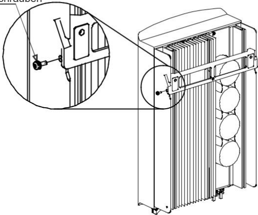
Abbildung 4.5 Wandhalterung
