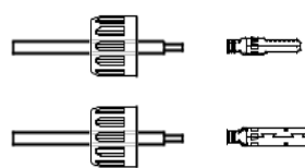
Abbildung 4.9 Einführen des Drahtes in die Steckverbinder-Überwurfmutter und Kontaktstift
