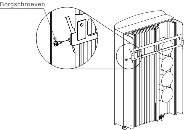
Figuur 4.5 wandmontagebeugel
