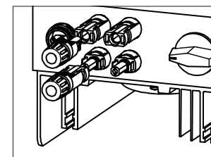
Figuur 4.12 Sluit de DC-connectoren aan op de omvormer
