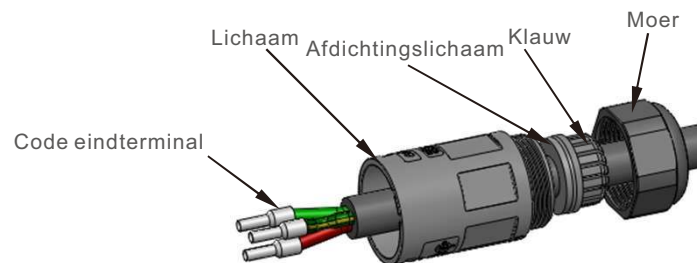
Figuur 4.14 AC-netterminalconnector
