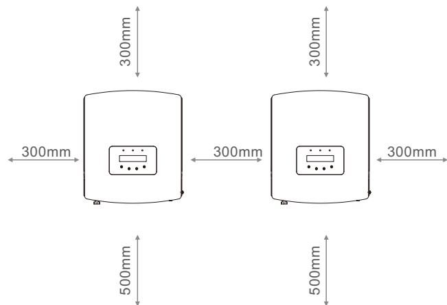
Figuur 4.2 Omvormer montagespeling
