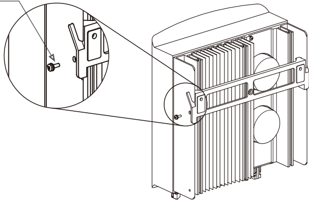
Figuur 4.5 wandmontagebeugel
