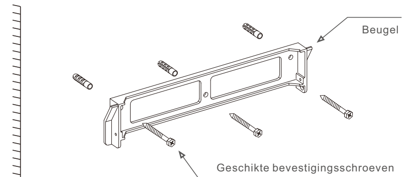
Figuur 4.4 Wandmontage van de omvormer
