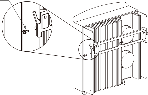
Figura 4.5 Staffa per montaggio a parete
