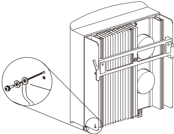
Figura 4.19 Collegare il conduttore di terra esterno
