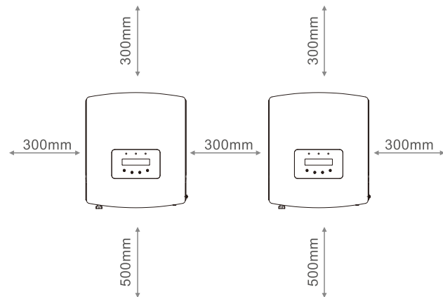
Figura 4.2 Distanza di montaggio dell'inverter
