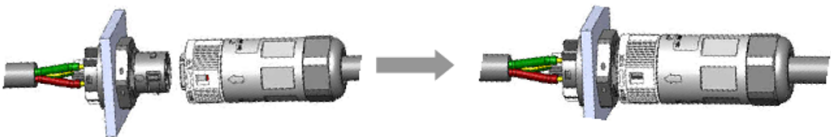
Figura 4.18 Connettere il Connettore AC all'inverter
