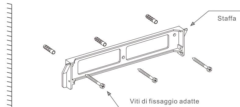
Figura 4.4 Montaggio a parete dell'inverter
