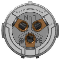
Figura 4.13 Connettore Terminale Griglia AC Interno
