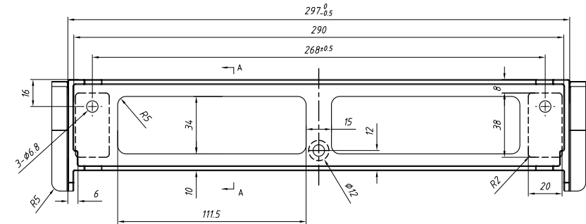
Figura 4.3 Montaggio a parete dell'inverter
