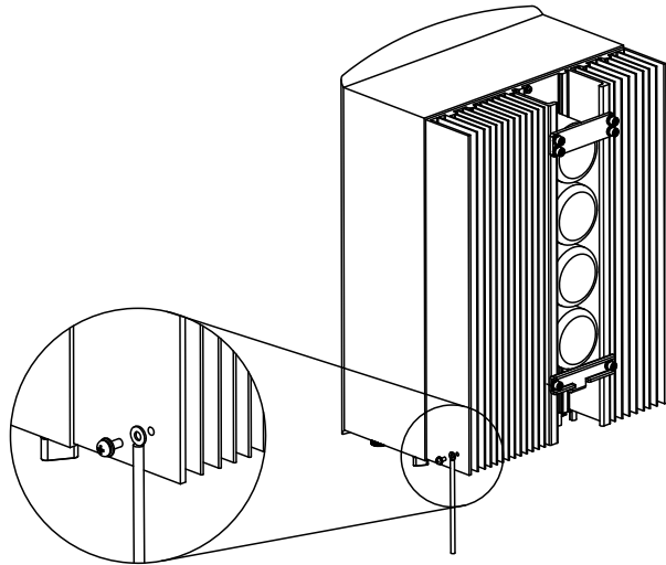
Abbildung 4.6 Anschluss des externen Erdungsleiters
