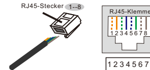
Abbildung 4.34 Abisolieren der Isolierschicht und Anschluss an RJ45-Stecker
