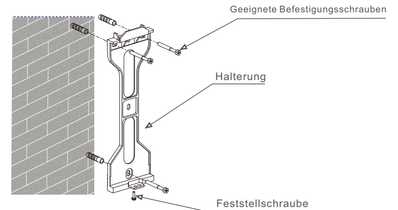
Abbildung 4.4 Befestigung der Halterung an der Wand
