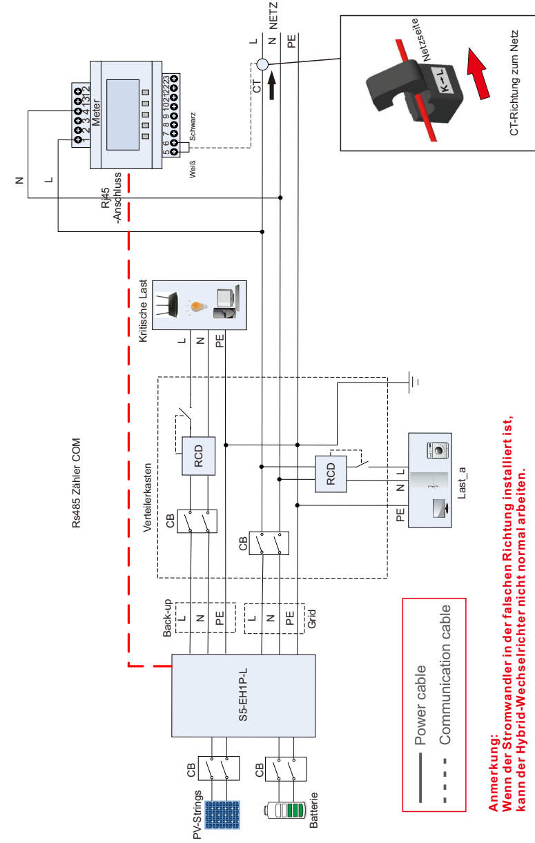
Abbildung 4.39 (AcrelACR10R-16DTE)
