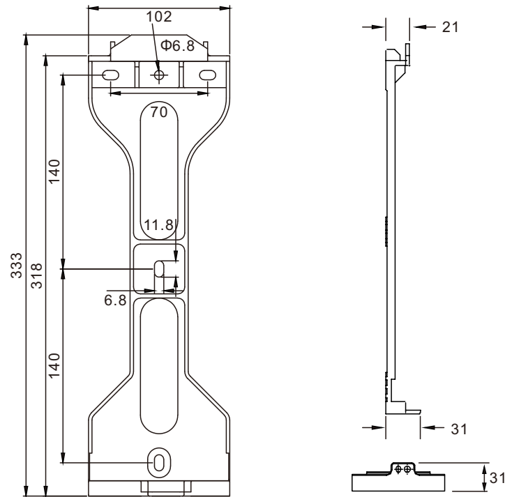
Abbildung 4.3 Wandmontage des Wechselrichters
