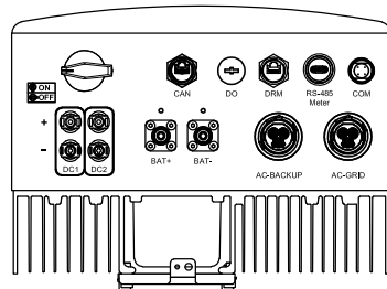
Abbildung 1.2 Seitenansicht von unten
