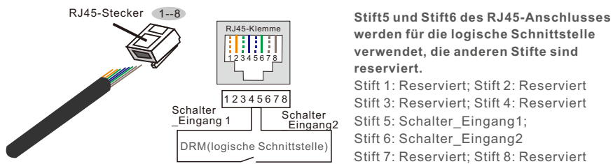
Abbildung 4.33 Abisolieren der Isolierschicht und Anschluss an RJ45-Stecker
