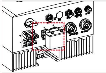
Abbildung 4.14 Installation der Klemmschutzabdeckung
